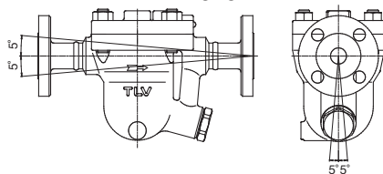
Schräglagentoleranz
