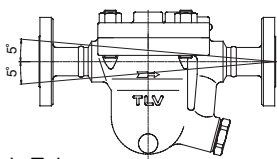
Horizontale Toleranz
