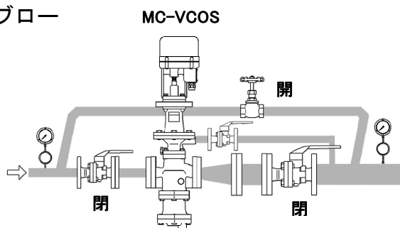
バイパス配管利用のブロー
