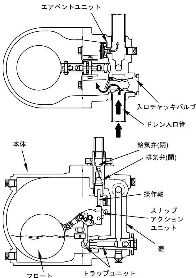
(1)、(3) ドレン流入工程 (排気工程)
