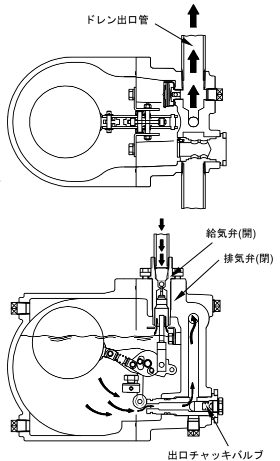
(2) ドレン圧送工程 (給気工程)
