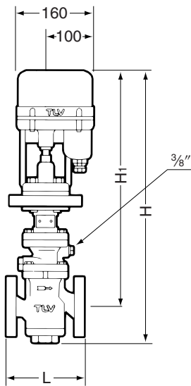
Abbildung zeigt DN 15 – 25. Formgebung von Ventilen größerer Nennweite weicht von der gezeigten etwas ab.
