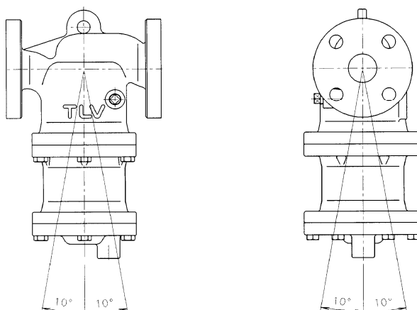
取付けの際の許容傾斜角度
