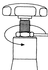
ロックナットをゆるめる
