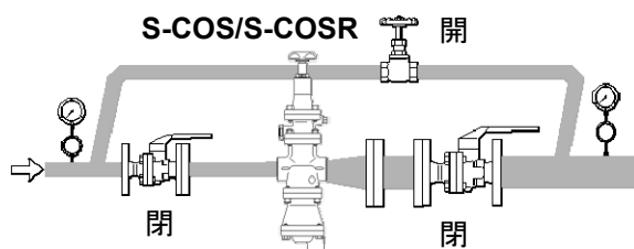
バイパス配管利用のブロー
