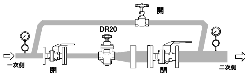
バイパス配管利用のブロー
