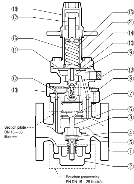
Section pilote
