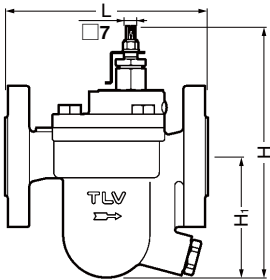
Bride de type DIN illustrée. La bride de type ASME est soudée au corps.
