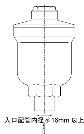
図3 (適切な配管部材の接続：VC2のみ)
