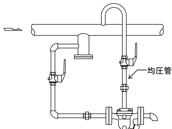
空気主管
