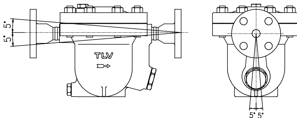
取り付けの際の許容傾斜角度
