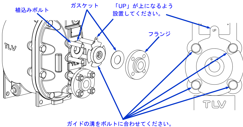
フランジレスチャッキバルブの取り付けについて (CKF5M)
