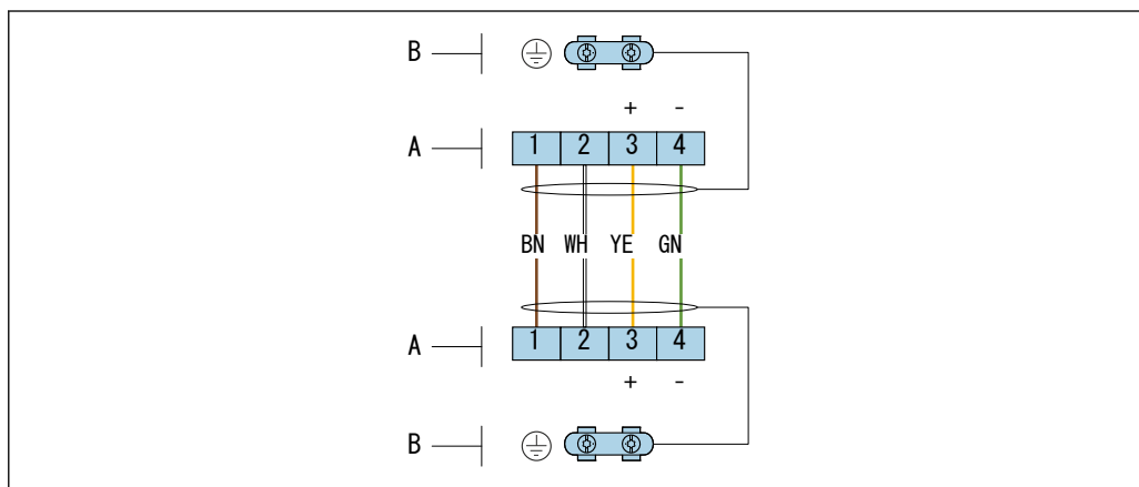
センサー接続ハウジングおよび変換器壁ホルダーの端子部の端子
