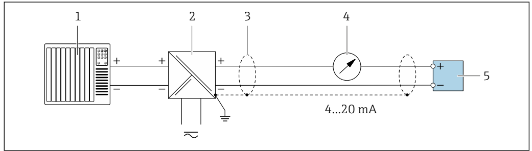
4~20mA電流出力（パッシブ）の接続例
