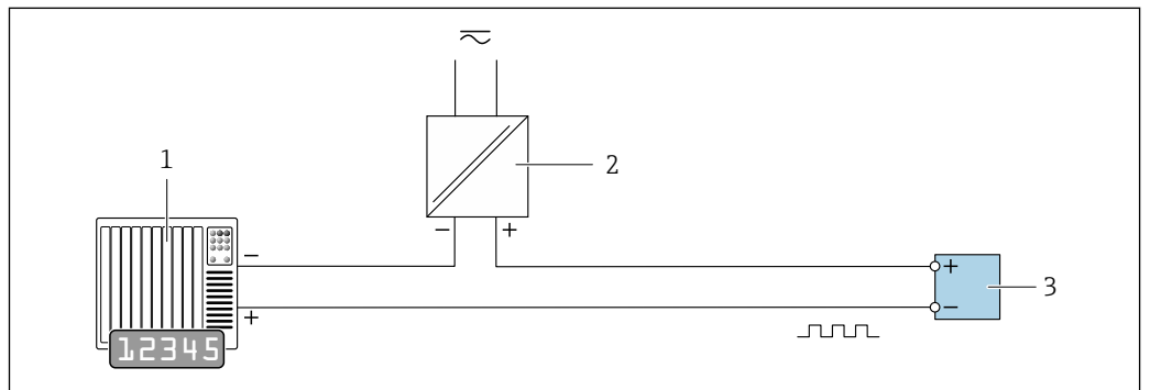
パルス/周波数出力（パッシブ）の接続例
