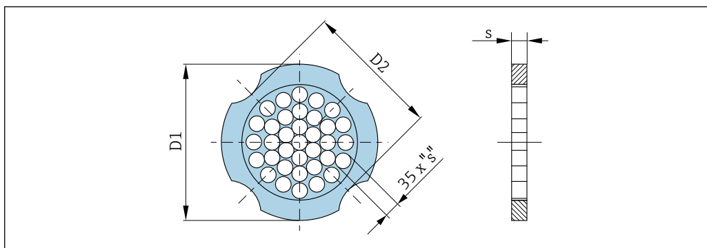
DIN EN 1092-1 : PN 10 準拠のフランジと組み合わせて使用 1.4404 (SUS 316 相当、SUS 316L 相当)
