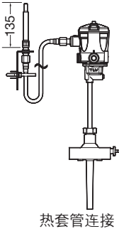
热套管连接
