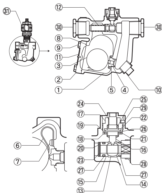
オリフィス部詳細
